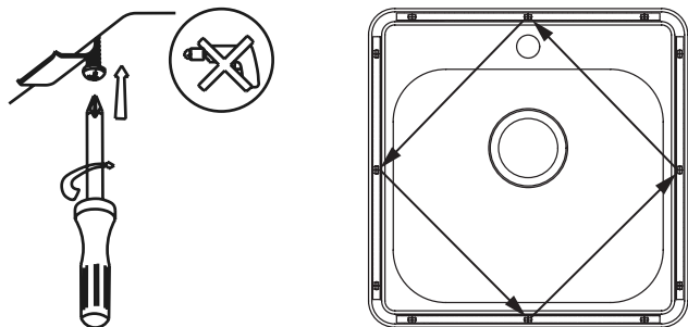
Схема затягивания
