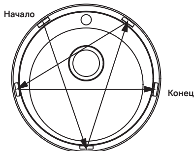
Схема затягивания
